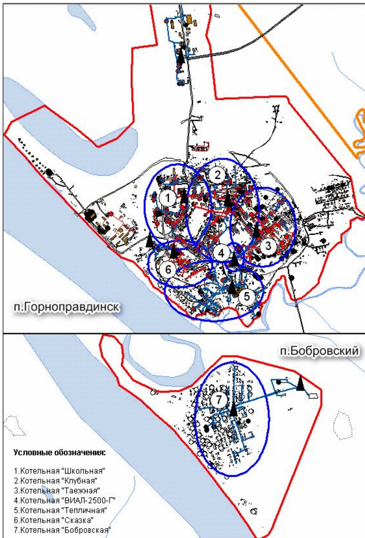
Рисунок 2.1 – Схема радиуса эффективного теплоснабжения теплоисточников с.п. Горноправдинск
